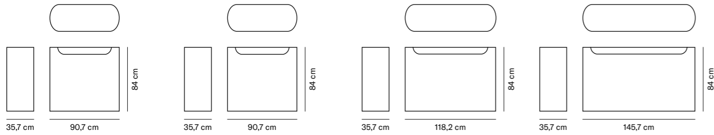
MEV-02-T Capacity: 226 L (2 x 113 L) NET: 32 kg | GROSS: 33 kg
