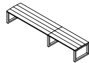
CET-23 300 x 61 x 46 cm NET: 64 kg | GROSS: 65 kg
